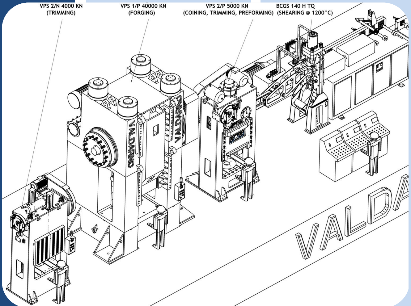
在4000吨机械式压机基础上的热锻压生产线
